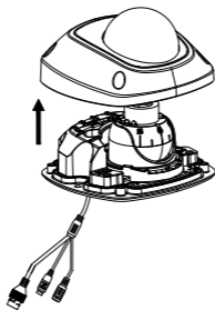
Рисунок 2-2 Демонтаж камеры
